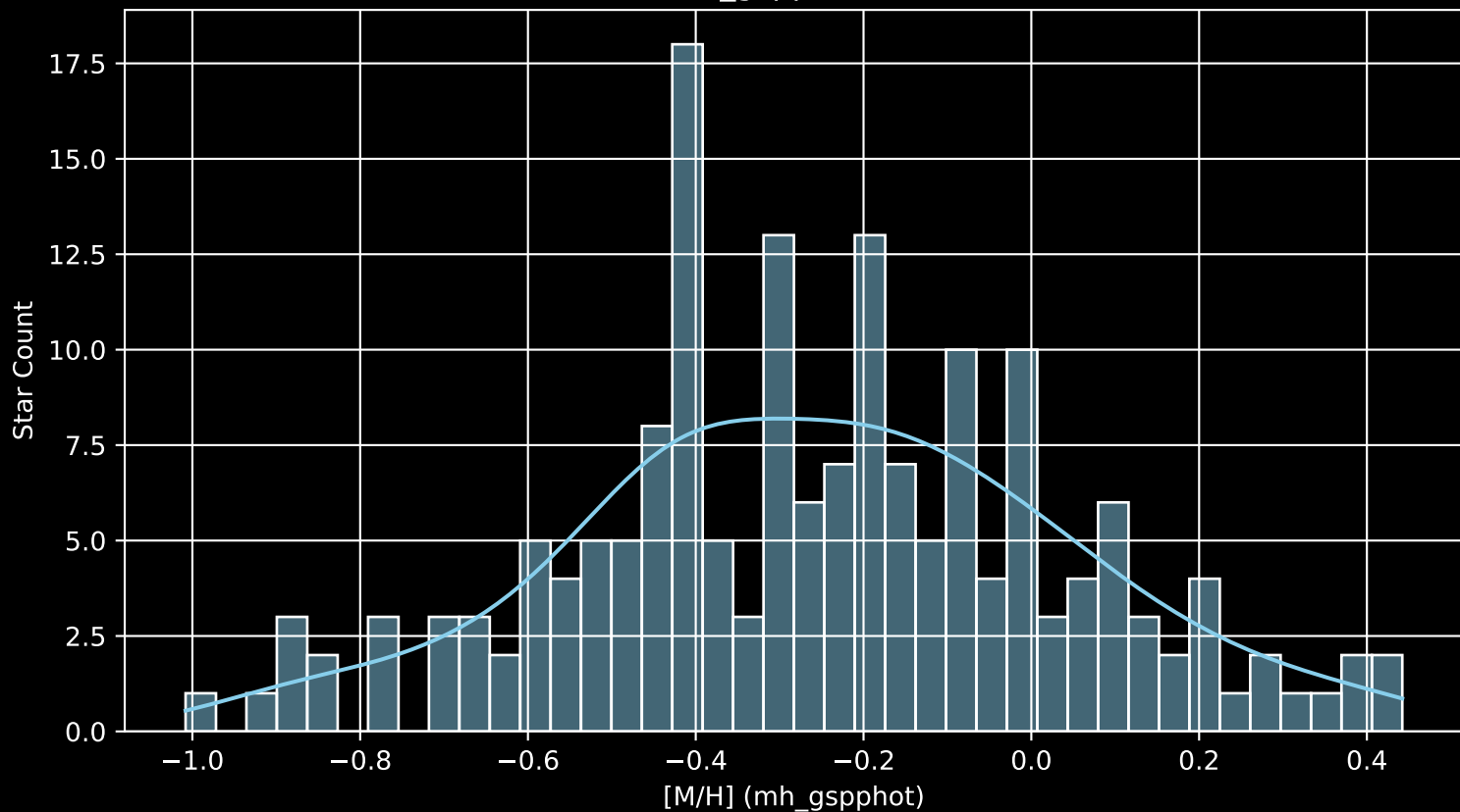
APOGEE DR17 Field: [159+39 MGA [M/H] (mh_gspphot) (n= 177)
